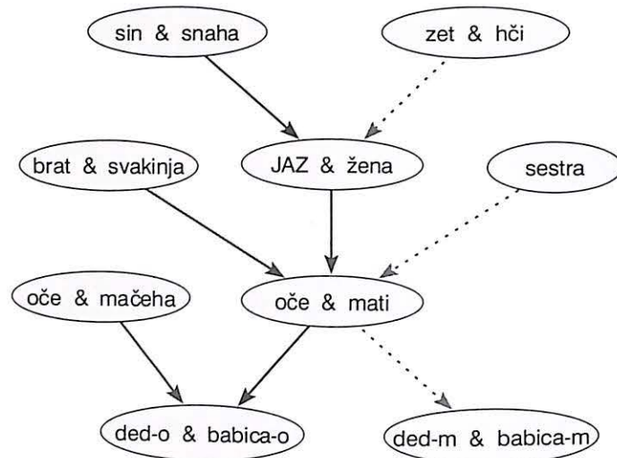
Slika 2: Parni rodovnik.
