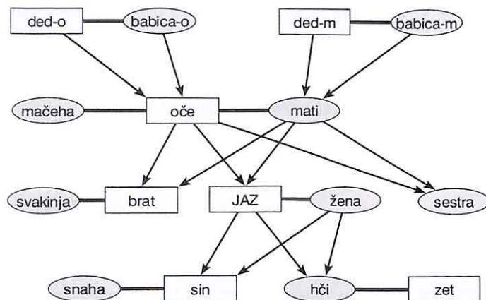
Slika 1: Navadni rodovnik.
